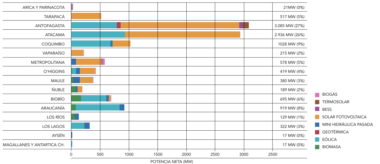
CAPACIDAD INSTALADA ERNC/ALMACENAMIENTO POR REGIÓN
