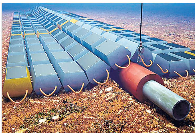
MANTAS de hormigón flexibles que se adaptan a la forma del ducto.
